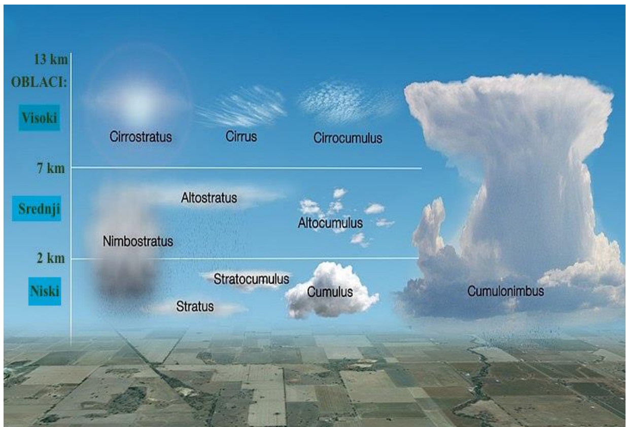
Sl. 9. Klasifikacija oblaka
