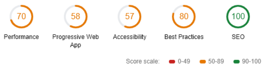
Slika 7. Lighthouse metrike
