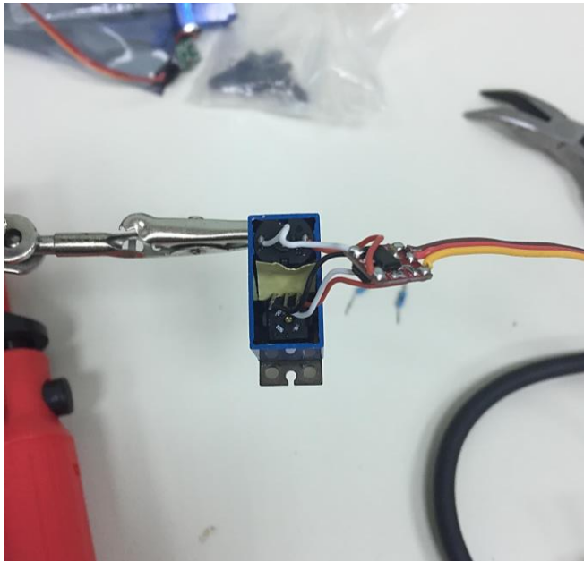
Slika 7.3 Rastavljanje TowerPro MG92B servomotor
