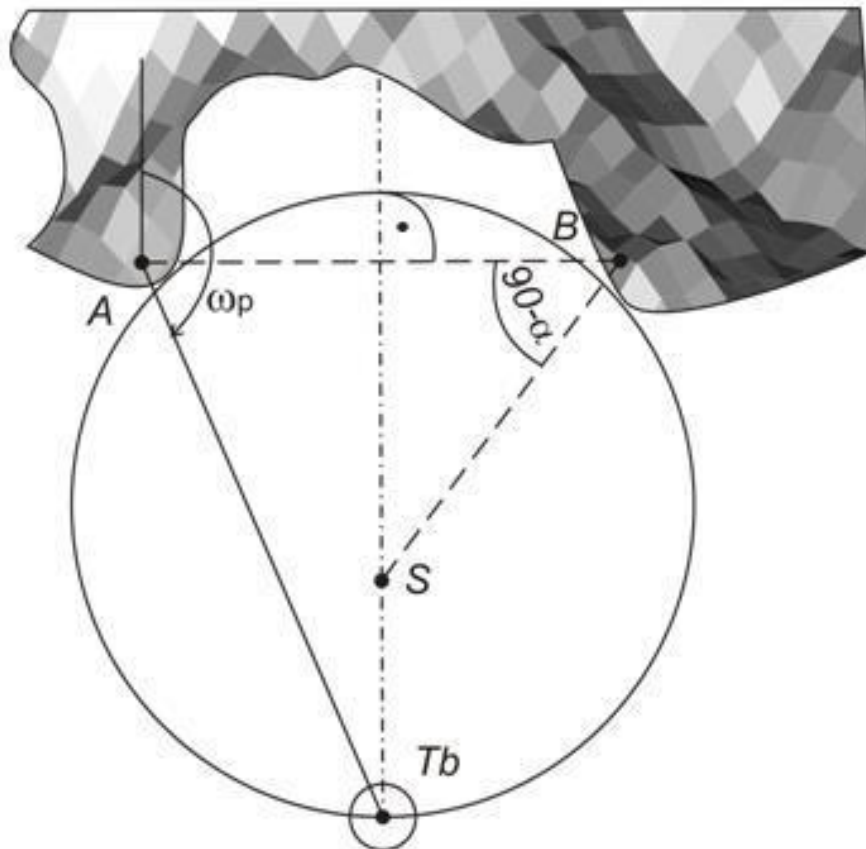
Slika 15. Pozicija određena pomoću azimuta i horizontalnog kuta [8]
