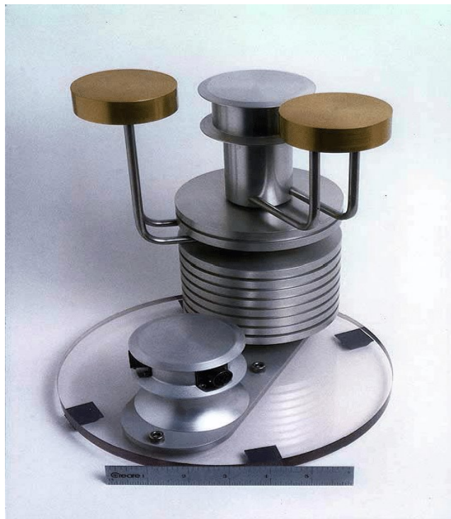
Slika 12. Minijaturni Braytonov hladnjak [25]
