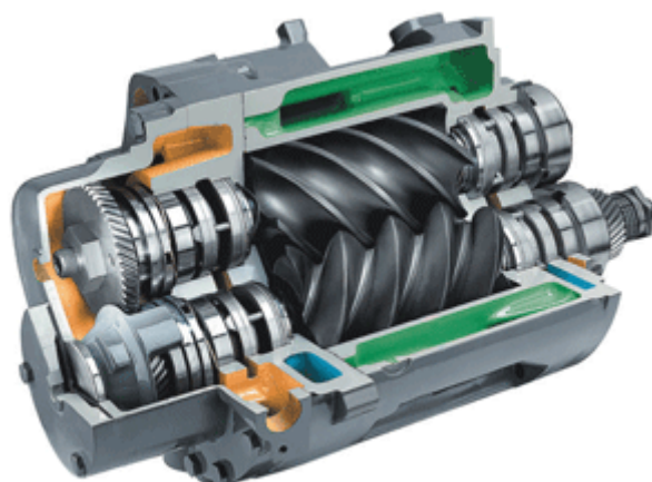
Slika 19. Vijčani kompresor[32]
