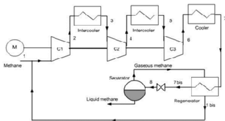
Slika 6. Shema Joule-Thomsonovog ciklusa[20]
