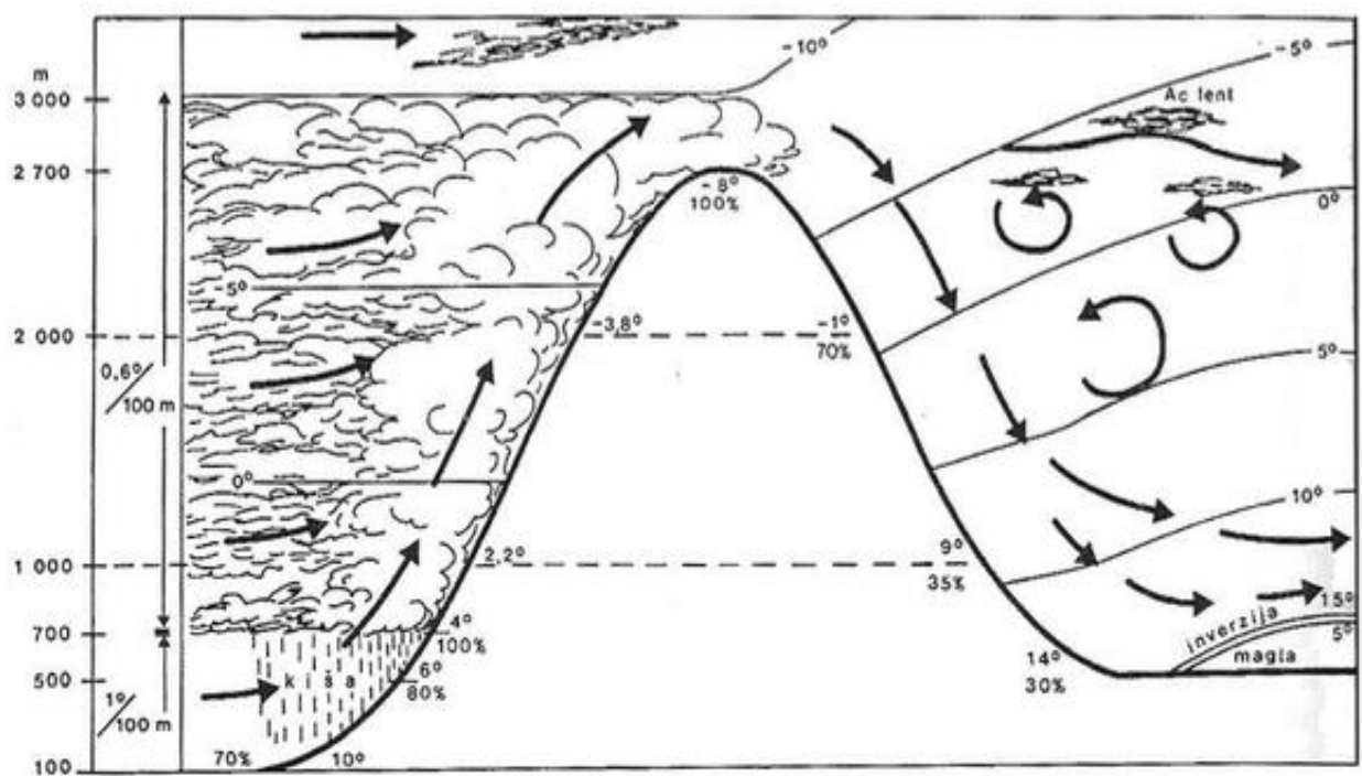
sl. 4. nastanak orogenetičkih oblaka
