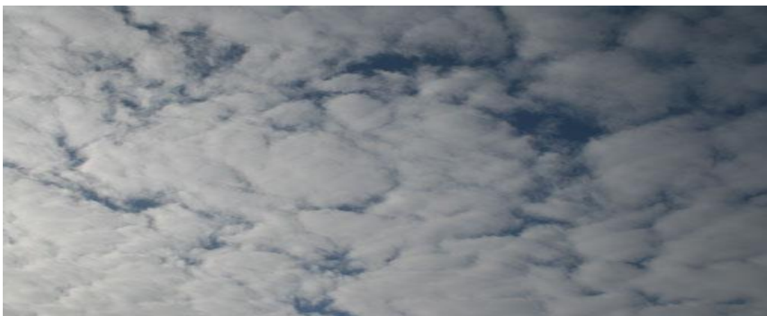
sl. 45. Perlucidus- Ova karakteristika se javlja kod Altocumulus-a, Stratocumulus-a.
