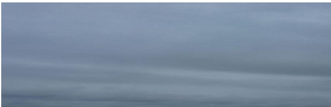
sl. 46. Opacus - Ova karakteristika se javlja kod Altocumulus-a, Altostratus-a, Stratocumulus-a i Stratus-a.
