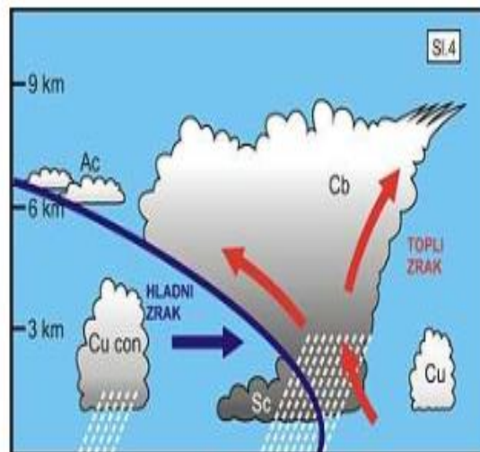
SI.4 Prikaz naoblake brze hladne fronte s nestabilnim toplim zrakom Ac - altokumulus Sc - stratokumulus Cb - kumulonimbus Cu - kumululus Cu con - kumululus kongestus
