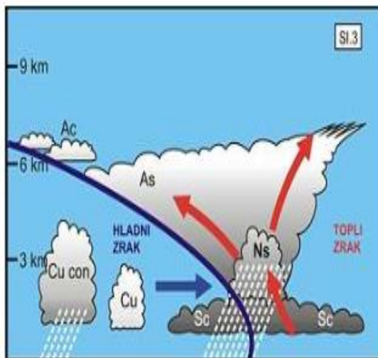
SI.3 Prikaz naoblake brze hladne fronte sa stabilnim toplim zrakom Ac - altokumulus Sc - stratokumulus As - altostratus Ns - nimbostratus Cu con - kumululus kongestus Cu - kumululus
