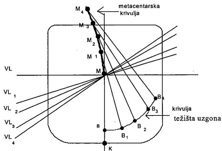
Slika 2: Krivulje težišta uzgona B i metacentra M [2]
