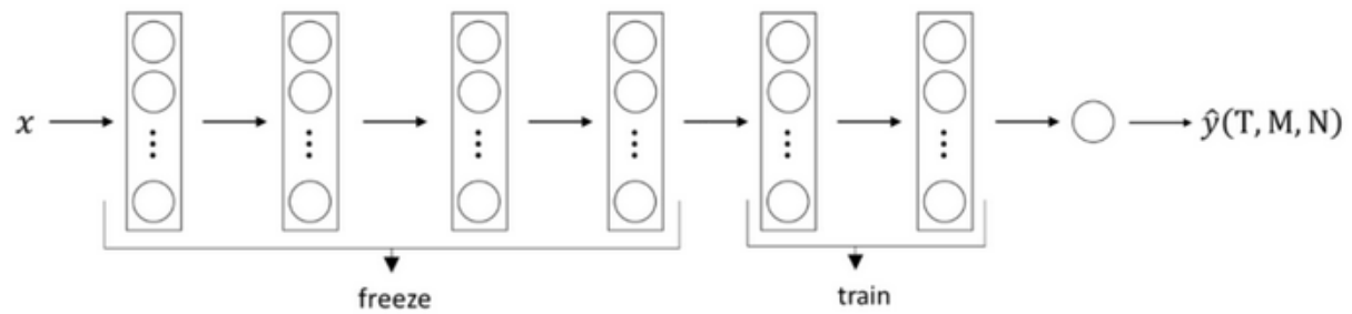
Slika 45 - Prijenosno učenje [33]
