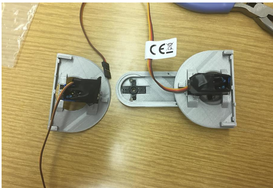
Slika 7.6 Instalacija križića i pogonskih servomotora na osovinu modula
