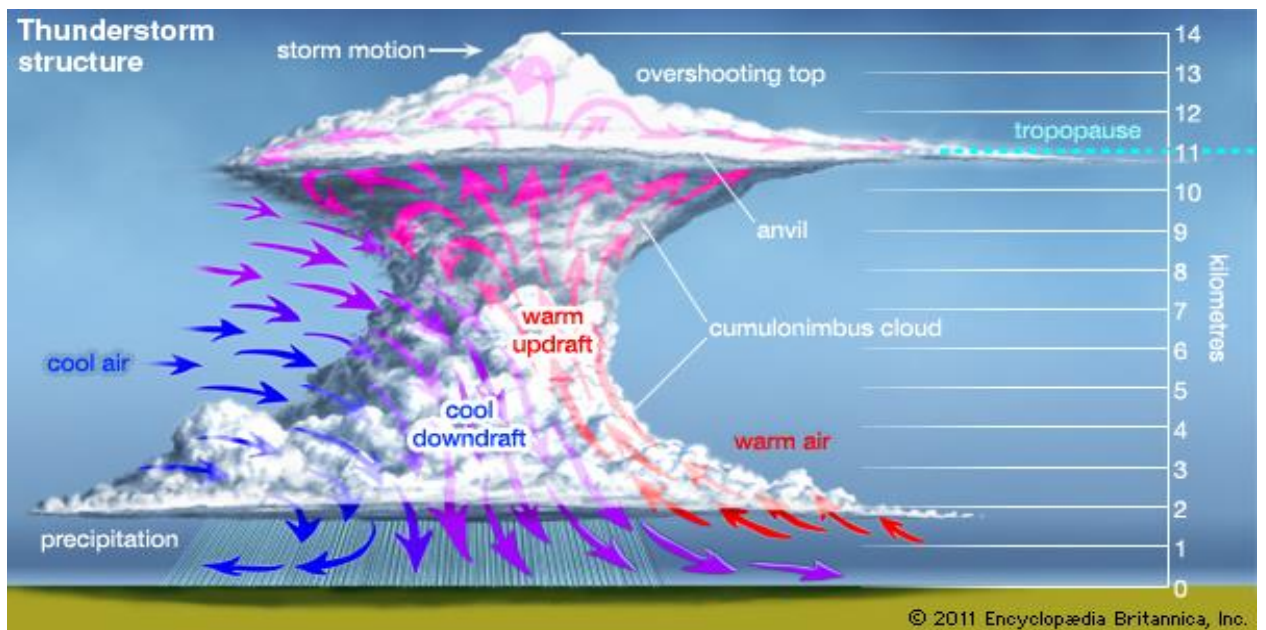
sl. 19. Cumulonimbus
