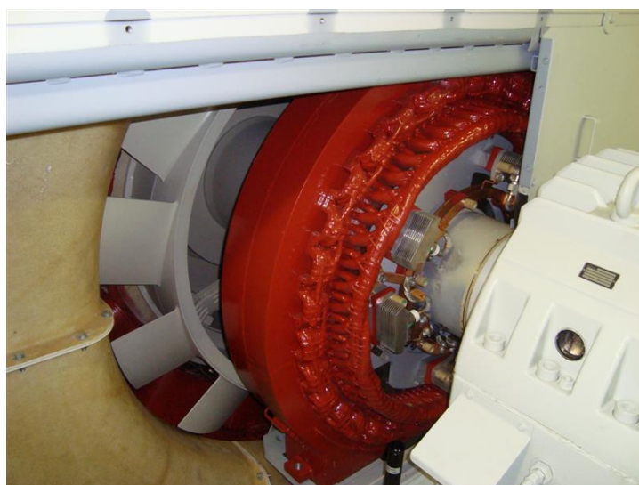
Slika 2.3: Uzbuđivanje sinkronog generatora
