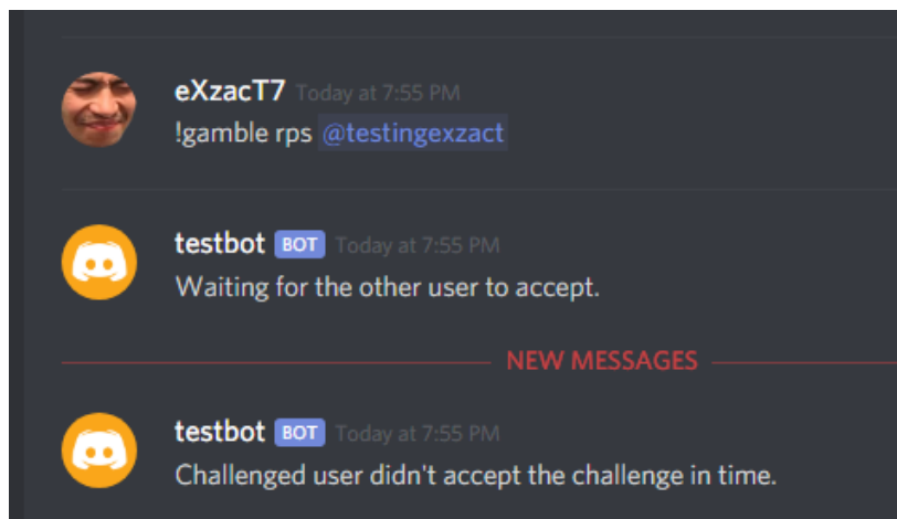
Slika 18 - Gamble naredba(1)
