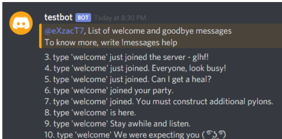
Slika 28- Messages naredba
