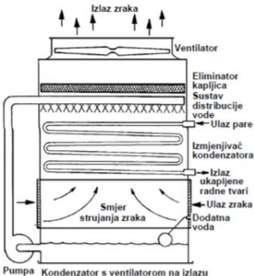
Slika 22. Evaporativni kondenzator [15]
