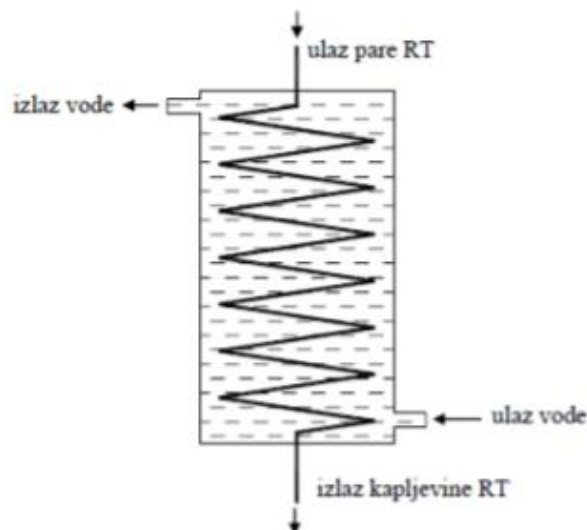
Slika 16. „Shell and coil“ kondenzator [2]
