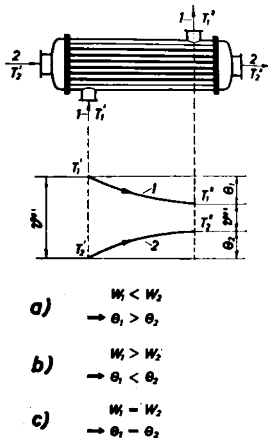
Slika 2. istosmjerni izmjenjivač topline [5]
