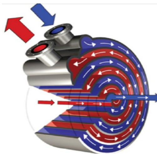
Slika 10. Spiralni pločasti izmjenjivač topline [10]
