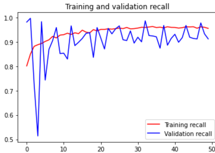
Slika 104 - Trening i validacijska odziv InceptionV3 modela
