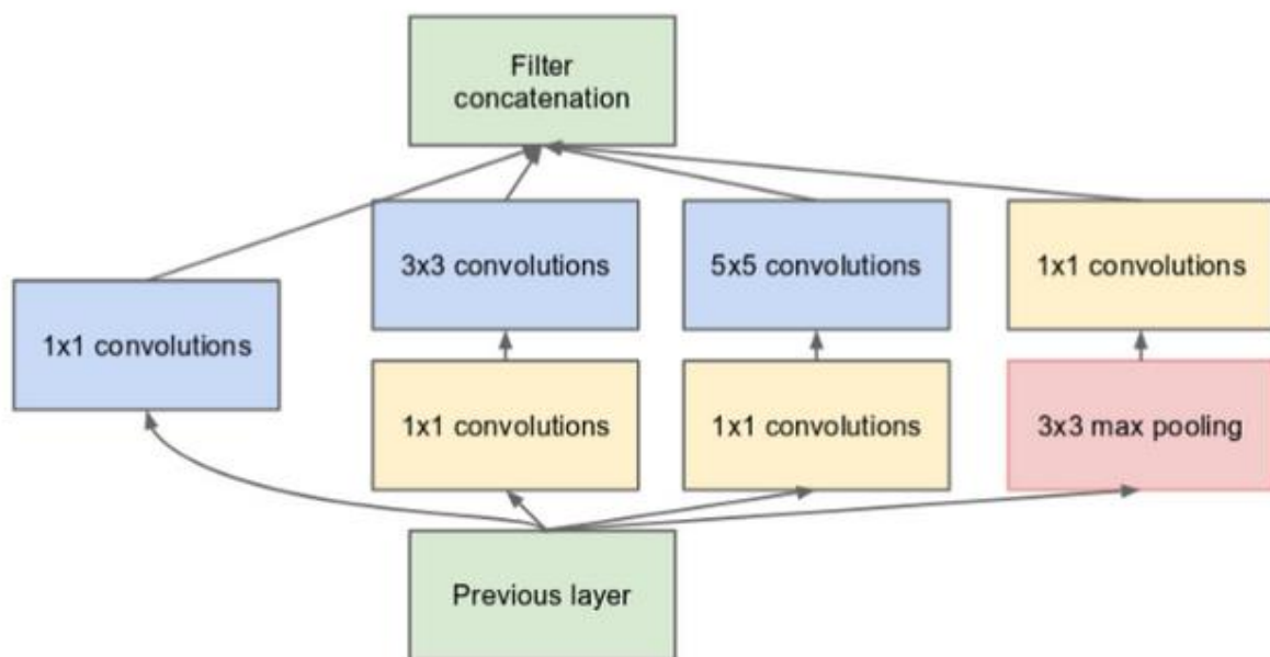
Slika 48 - Inception modul s 1x1 konvolucijama [34]
