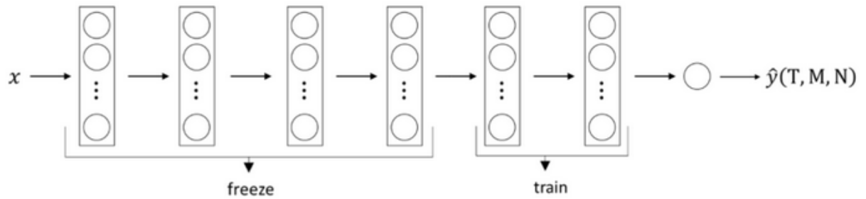
Slika 45 - Prijenosno učenje [33]
