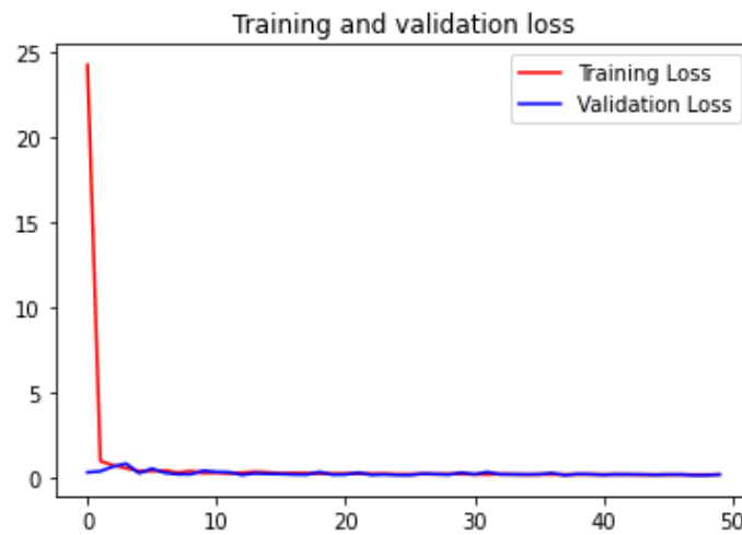
Slika 105 - Trening i validacijski gubitak InceptionV3 modela
