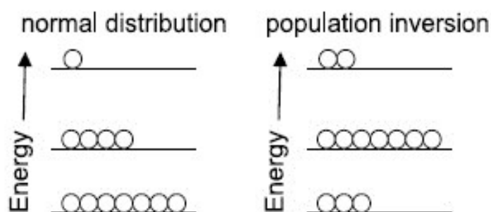
Slika 9. Inverzija populacije
