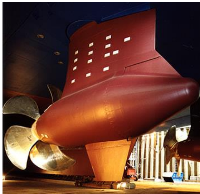
Slika 13. Azipod
