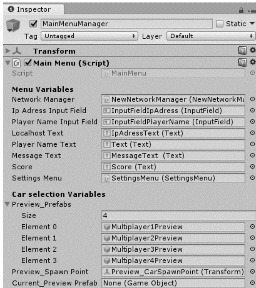
Slika 41. MainMenuManager
