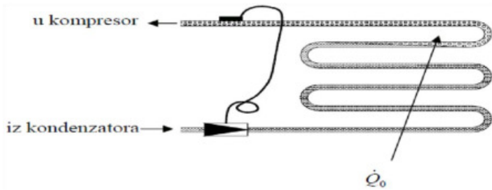
Slika 19. Suhi isparivač
