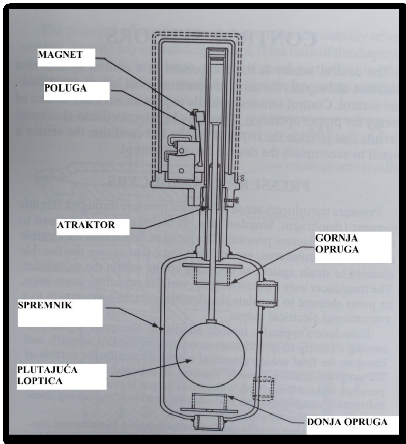
Slika 12. Shema prekidača s plovkom [12]
