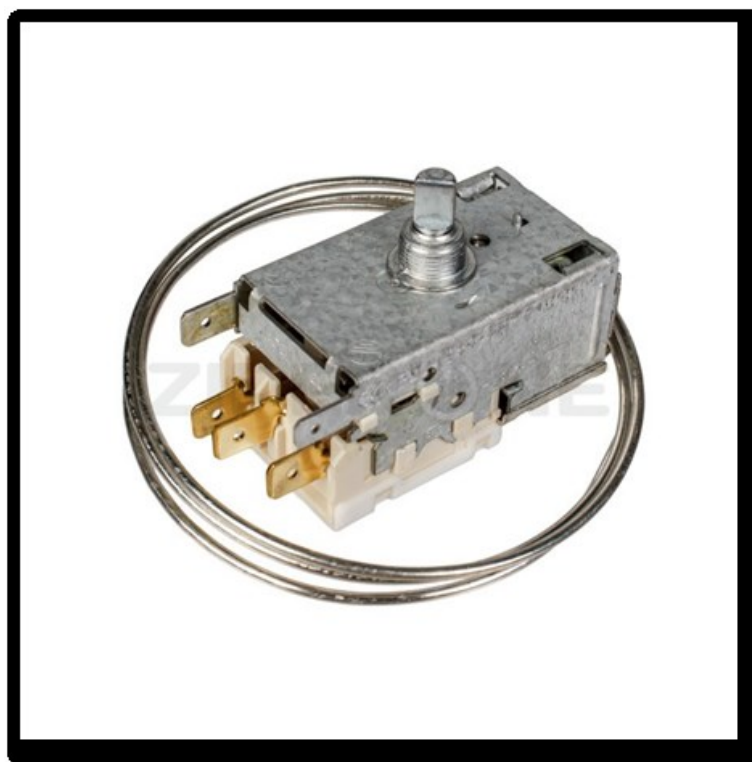
Slika 9. Indirektni termostat [9]
